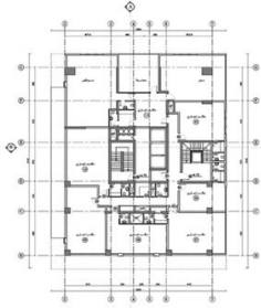
مسقط الطابق الاول
